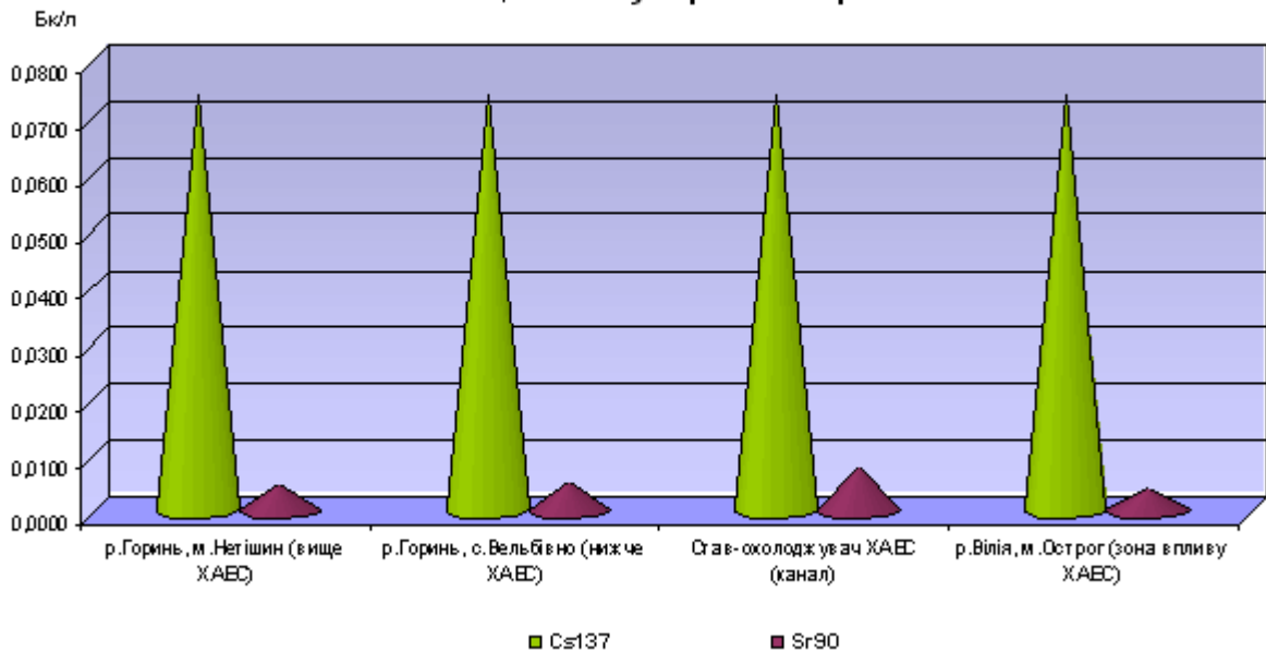
Рис. 11. Радіоактивне забруднення поверхневих вод у зоні впливу Хмельницької АЕС у вересні 2016 р.
