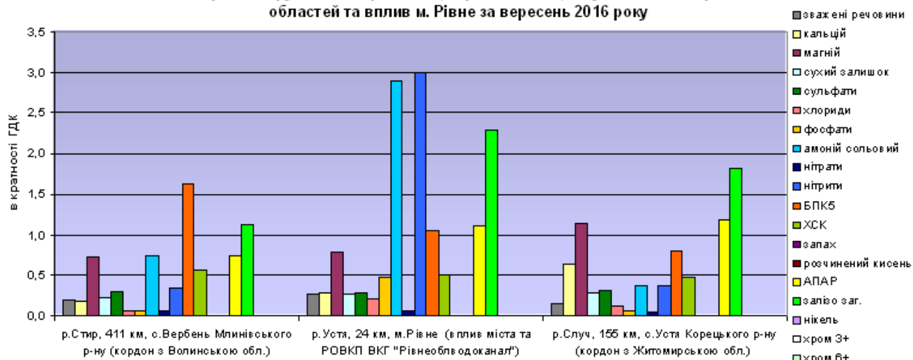
Рис. 7. Концентрації забруднюючих речовин (в кратності ГДК) в пунктах спостережень на межі областей та впливу м. Рівне за вересень 2016 року
