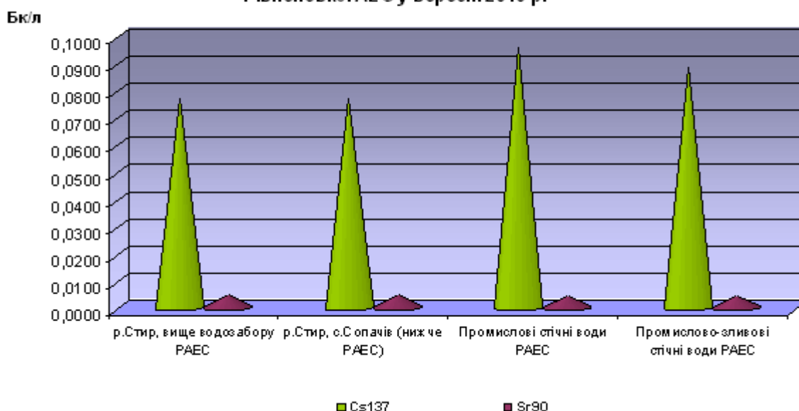
Рис. 10. Радіоактивне забруднення поверхневих вод у зоні впливу Рівненської АЕС у вересні 2016 р.
